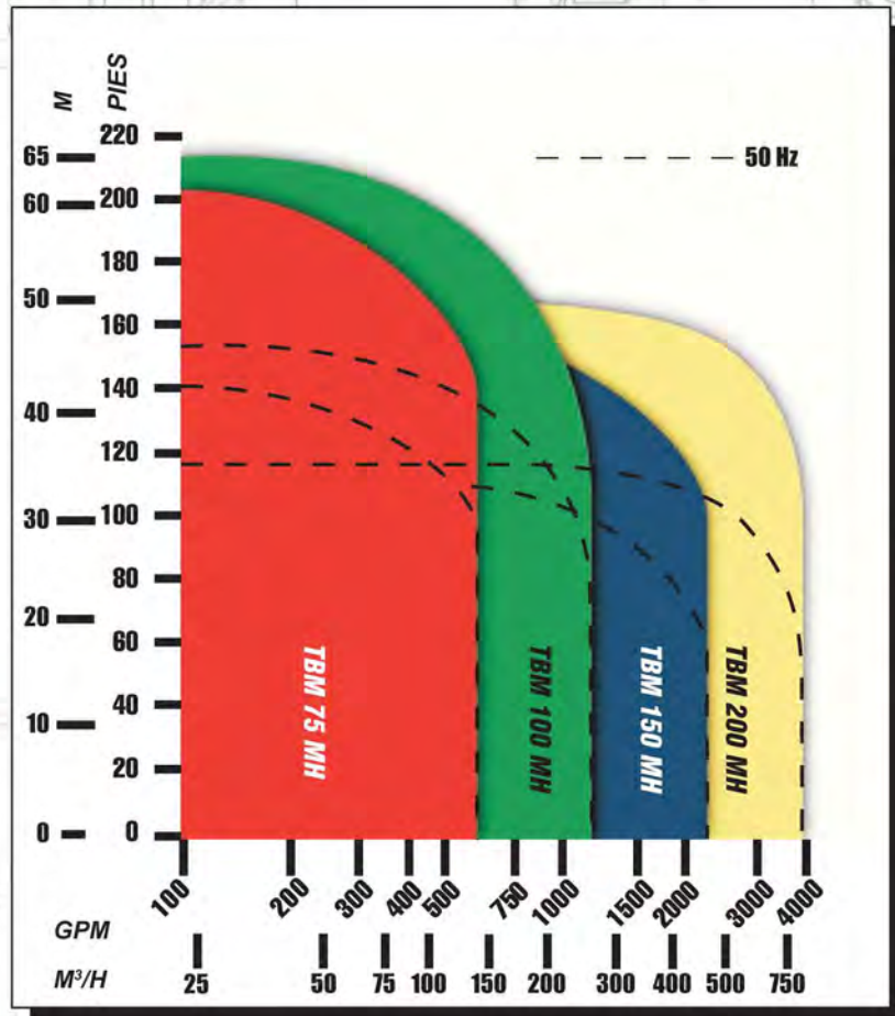
BOMBA MODELO TBM200MH-PBO CON OPCIONES DE CAMISAS DE ENFRÍAMIENTO (AGUA) Y ANILLO DE CHORROS A PRESION
